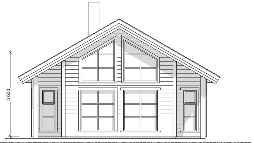
Fasade 4
