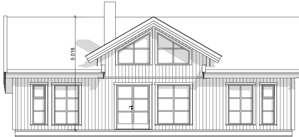
Fasade 3
